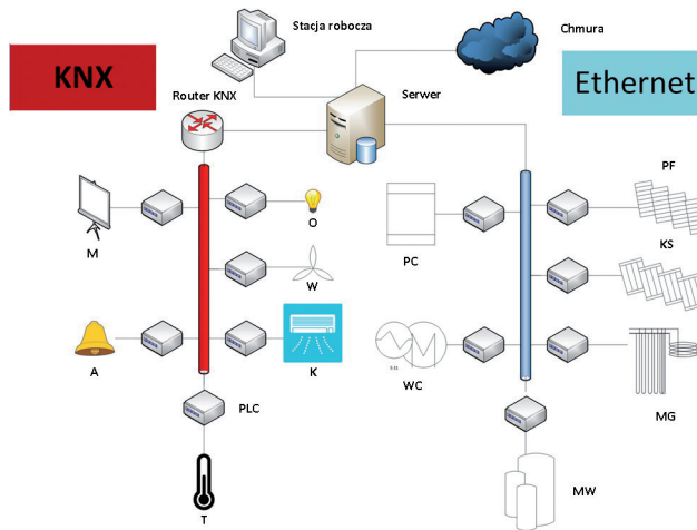
Ryc. 8. Schemat poglądowy instalacji akwizycji danych
